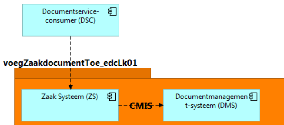
Figuur 20: Flow Voeg Zaakdocument toe
